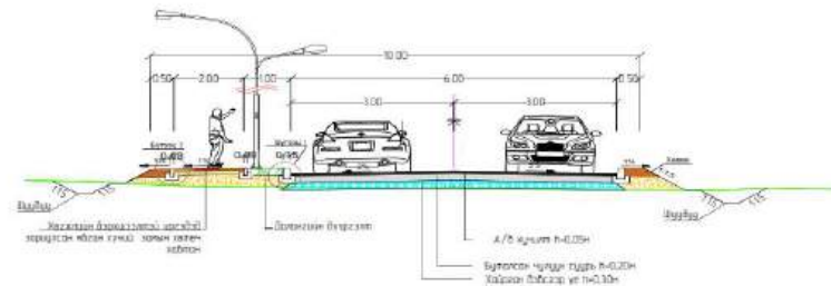
АВТО ЗАМЫН НЭГ МАЯГЫН ХӨНДЛӨН ОГТЛОЛ
