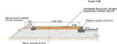
ЯВГАН ЗАМЫН ХУЧИЛТЫН ХИЙЦ
