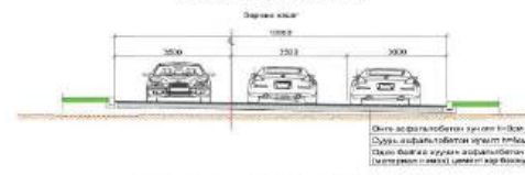
ЗАМЫН НЭГ МАЯГИЙН ХӨНДЛӨН ОГТЛОЛ-2 1-р хэсэг Km 0+240-Km 0+543.3
