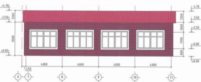
НҮҮРЭН ТАЛЫН БАЙГУУЛАЛТ / 6-11 ТЭНХЛЭГ / М1:100
